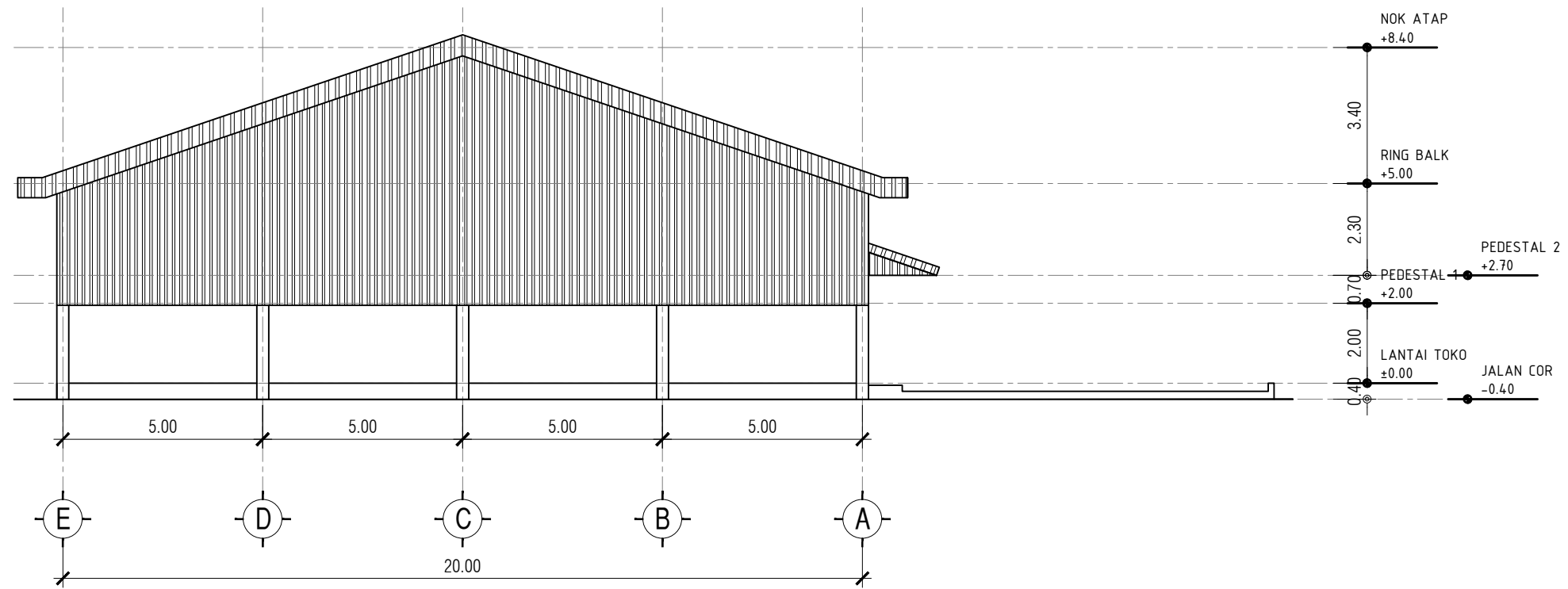
01 TAMPAK SAMPING KANAN KMP.A.01.04 SKALA 1 : 150
