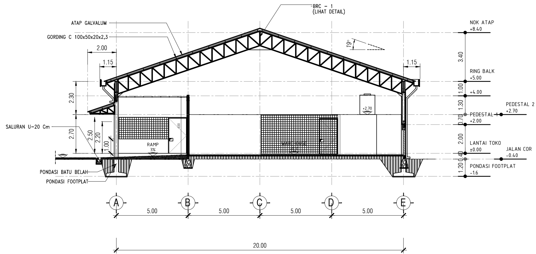
01 POTONGAN 6-6 KMP.A.01.07 SKALA 1 : 150
