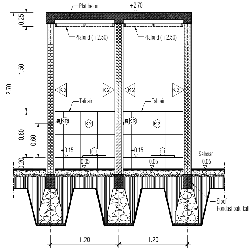
01 POTONGAN 1 - 1 KMP.A.01.16 SKALA 1 : 40
