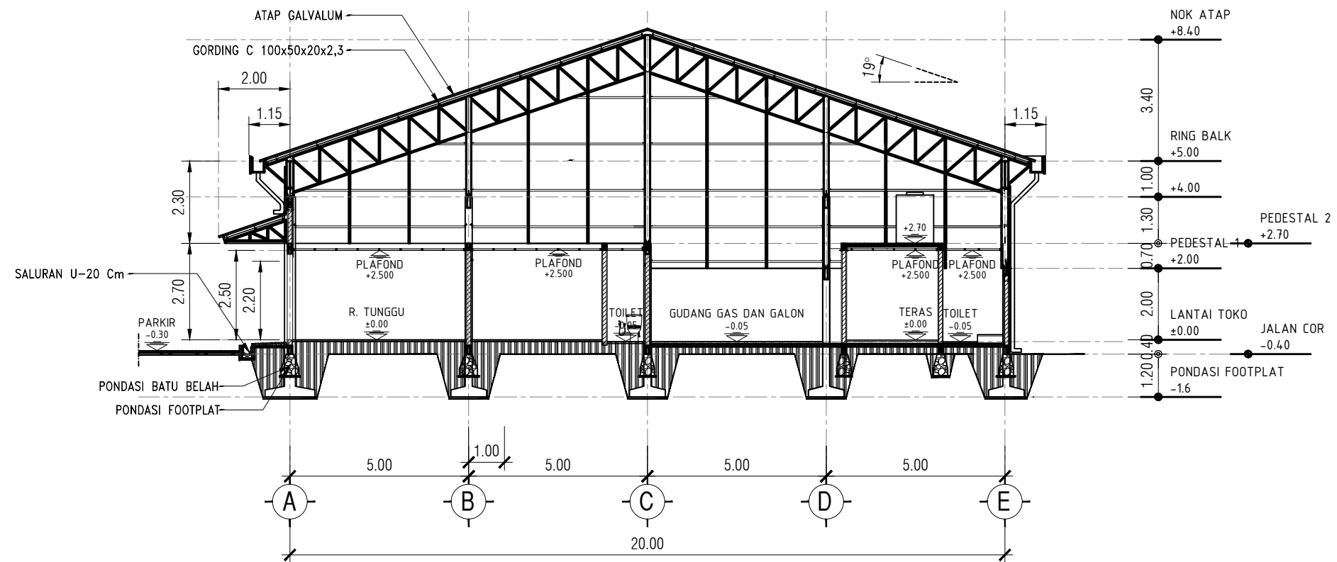
01 POTONGAN 4 - 4 KMP.A.0107 SKALA 1 : 150
