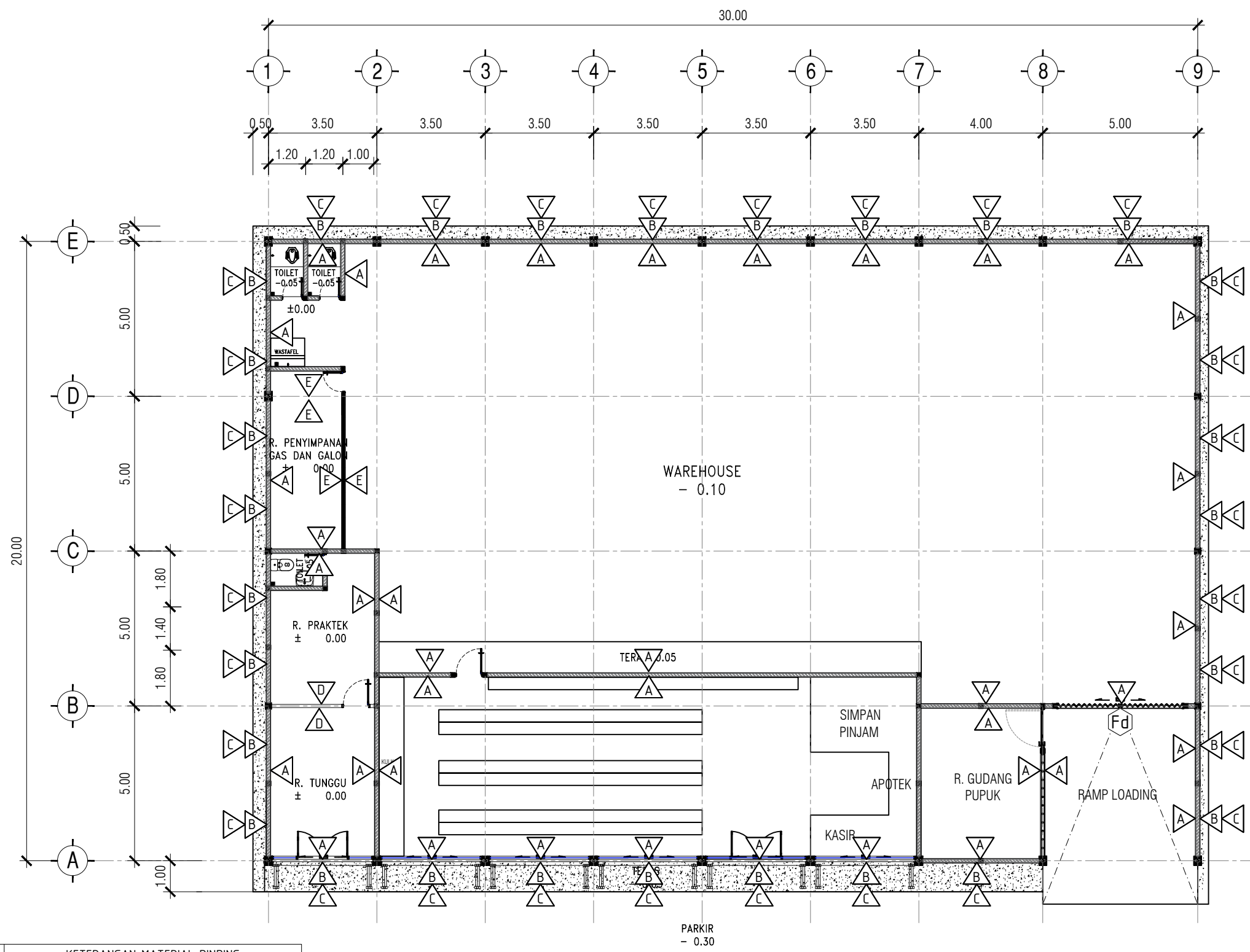
01 DENAH MATERIAL DINDING KMP.A.01.13 SKALA 1 : 150
