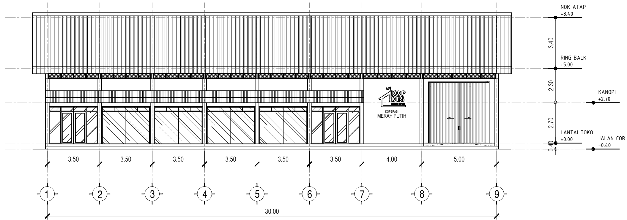
01 TAMPAK DEPAN KMP.A.0103 SKALA 1 : 150
