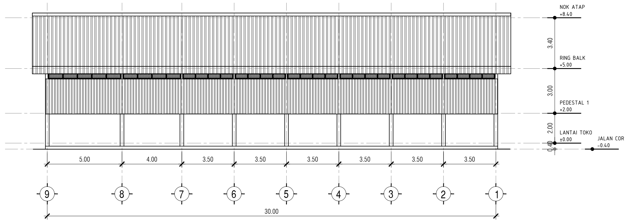
01 TAMPAK BELAKANG KMP.A.0103 SKALA 1 : 150
