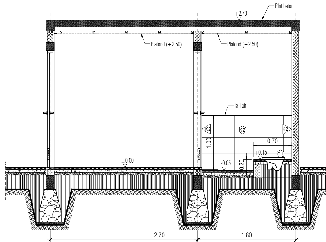
01 POTONGAN 2 - 2 KMP.A.01.16 SKALA 1 : 40
