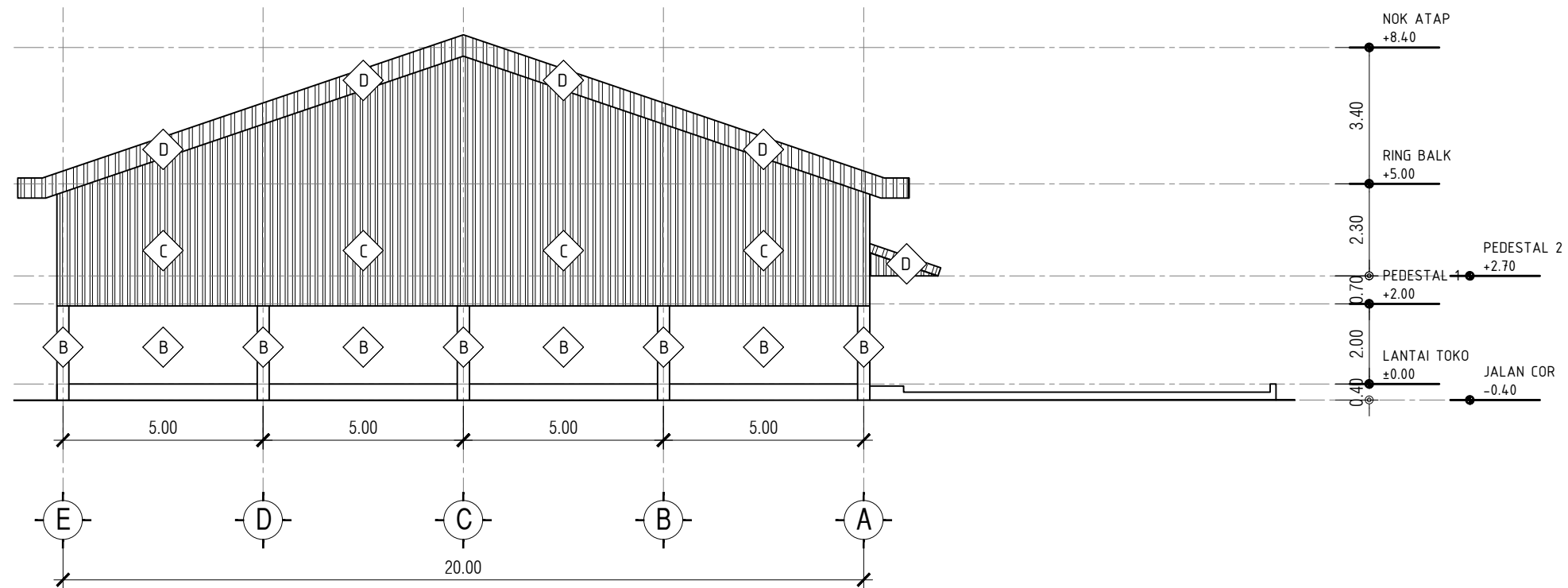
01 MATERIAL TAMPAK SAMPING KANAN KMP.A.01.15 SKALA 1 : 150
