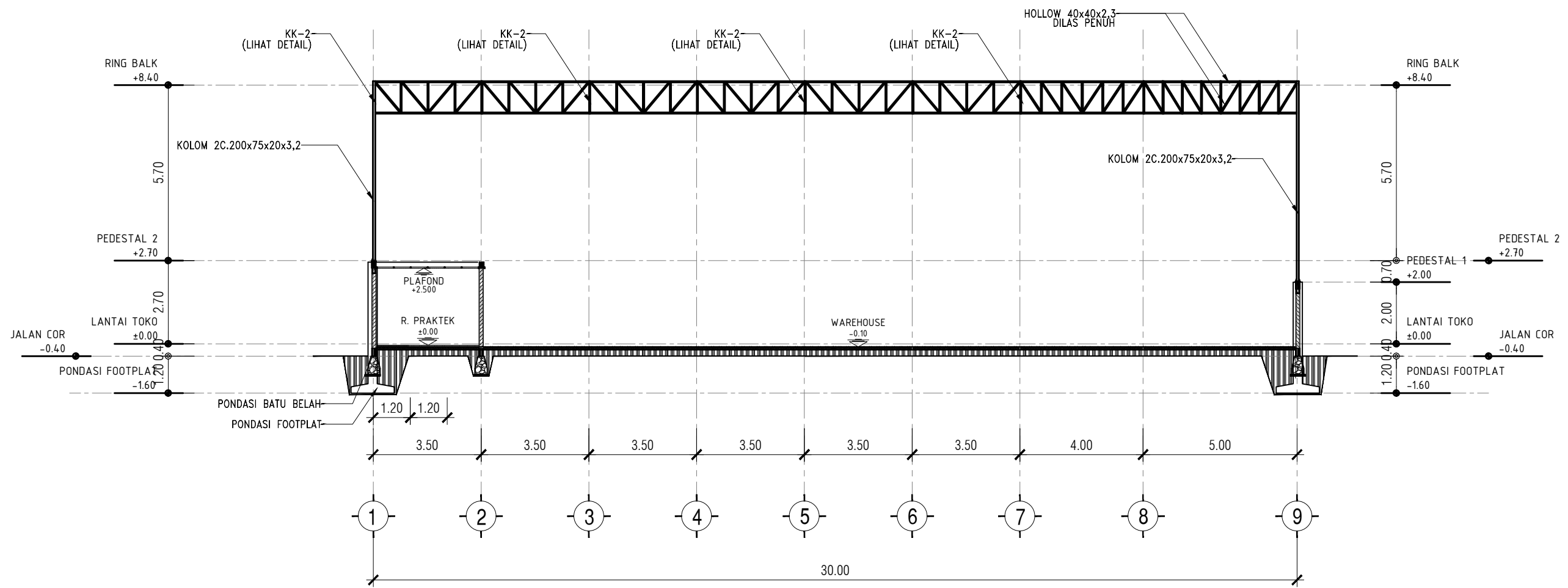
01 POTONGAN 3 - 3 KMP.A.01.06 SKALA 1 : 150
