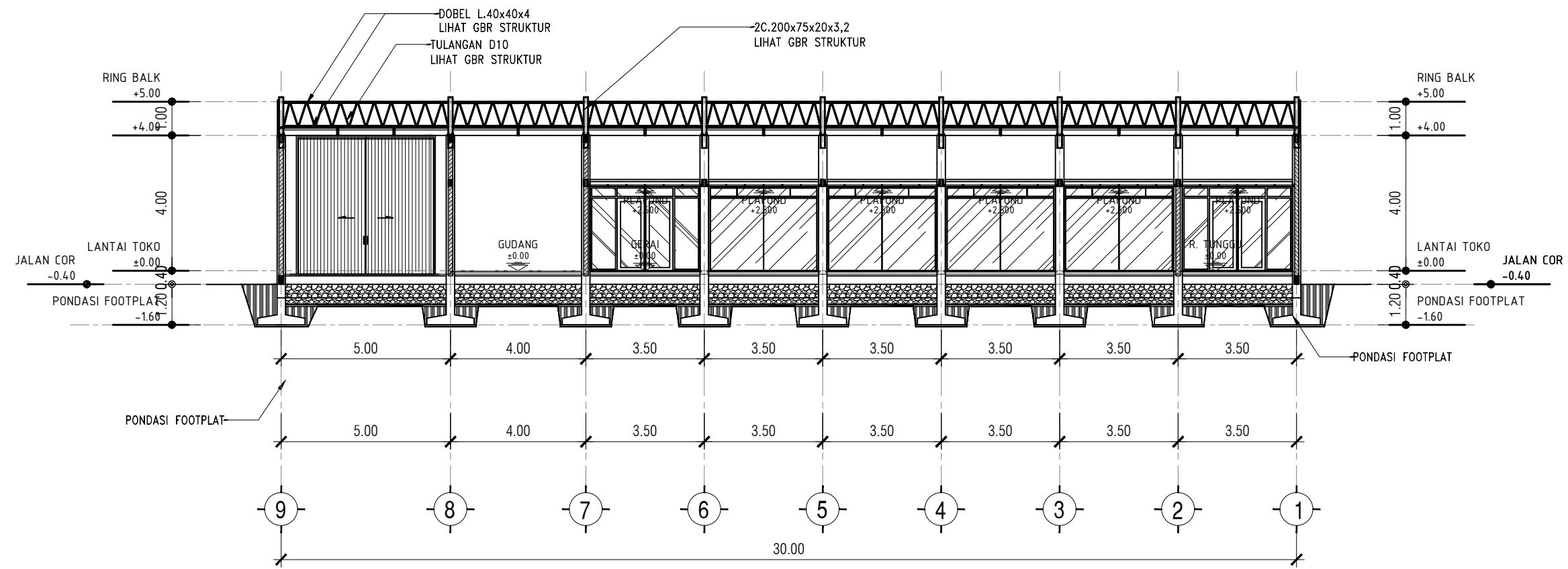
01 POTONGAN 1 - 1 SKALA 1 : 150
