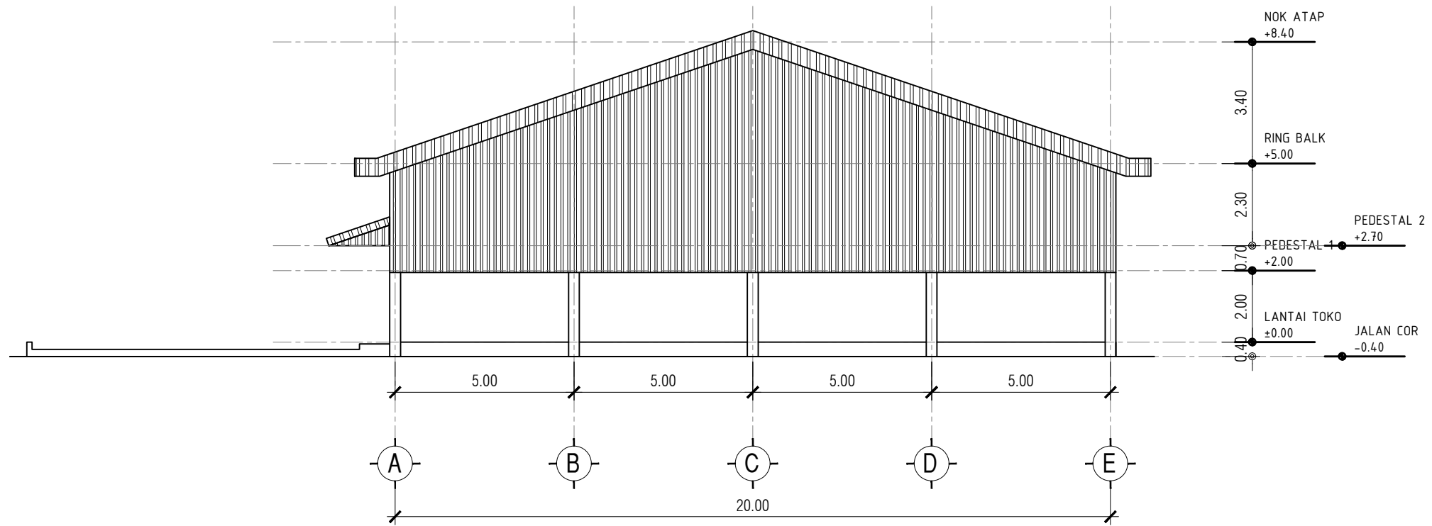
01 TAMPAK SAMPING KIRI KMP.A.01.04 SKALA 1 : 150
