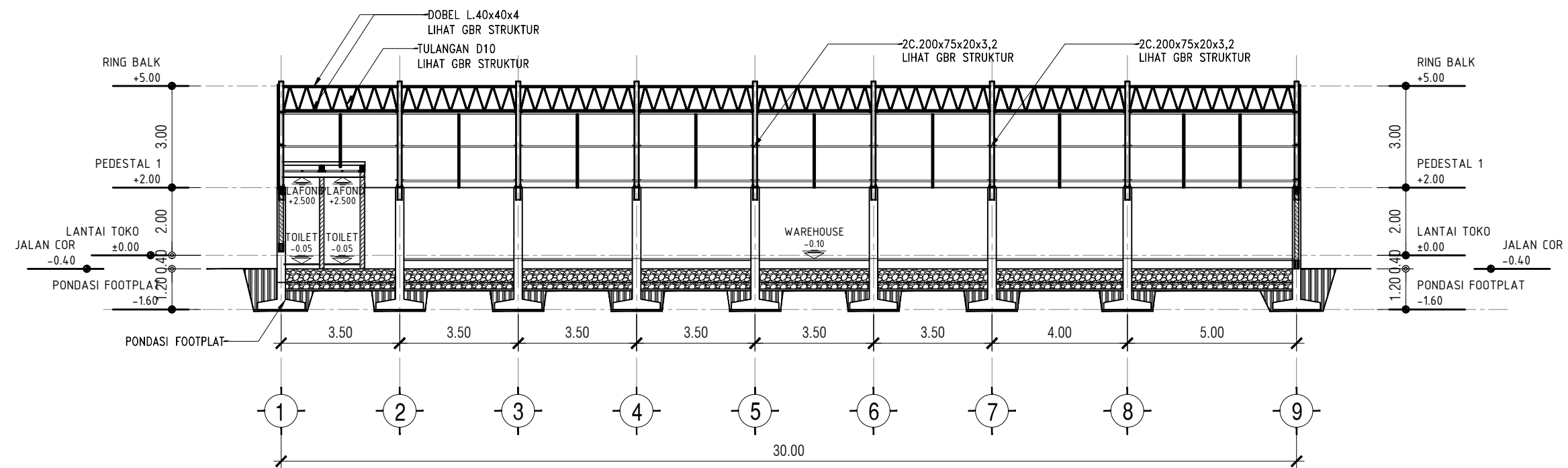
01 POTONGAN 1 - 1 SKALA 1 : 150
