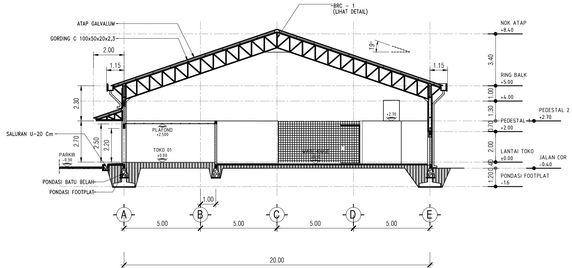
01 POTONGAN 5 - 5 KMP.A.0107 SKALA 1 : 150
