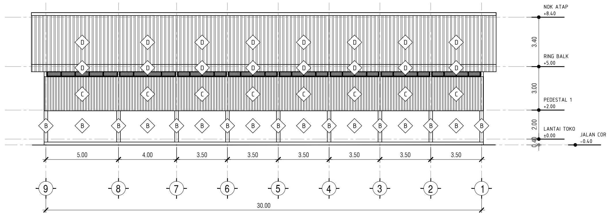
01 MATERIAL TAMPAK BELAKANG KMP.A.0114 SKALA 1 : 150
